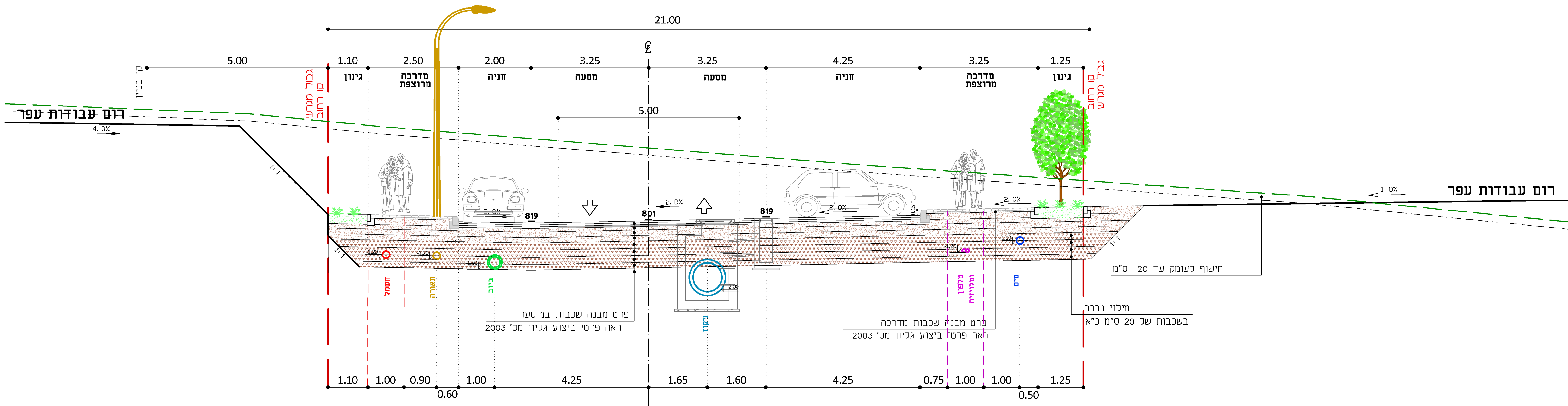
חתך טיפוסי כביש מס' 2 ברוחב 21 מ' חתכים : 208 - 233
