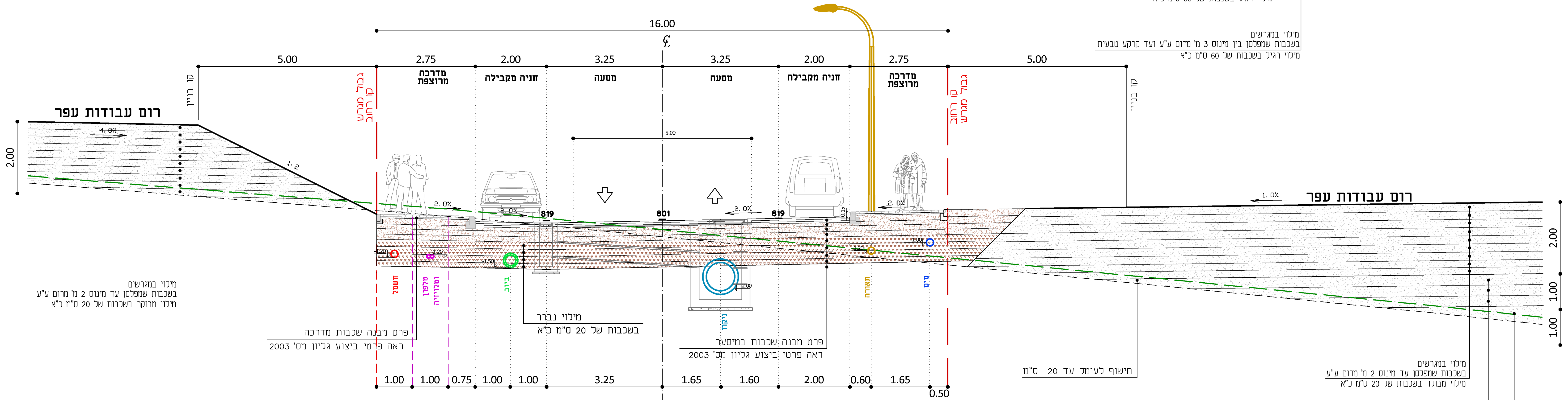
חתך טיפוסי כביש מס' 22 ברוחב 16 מ' בין חתכים : 2225 - 2205
