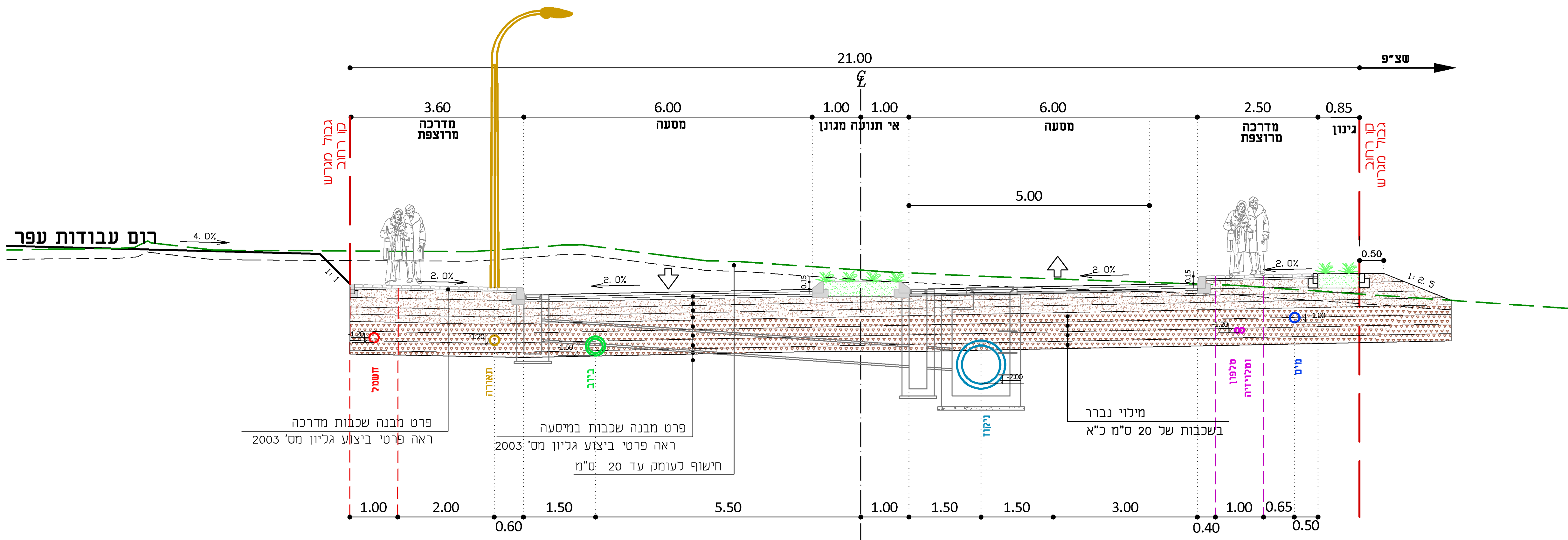
חתך טיפוסי כביש מס' 2 ברוחב 21 מ' חתכים : 208 - 206
